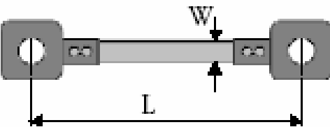
Rame (piastra di stagno) Copper (tin plate) NON RACCOMANDATA NOT RECOMMENDED
