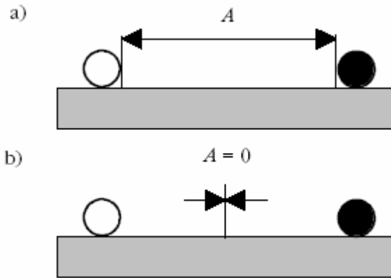
Esempi di cavi di potenza e cavi per la tecnologia dell'informazione che corrono paralleli senza divisore
