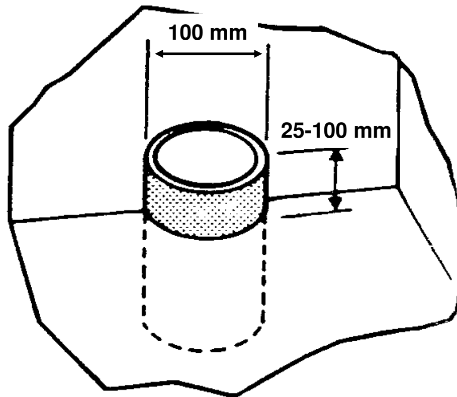
Manicotto
